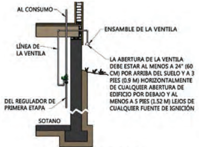
Figura 4: Instalación en un sótano
