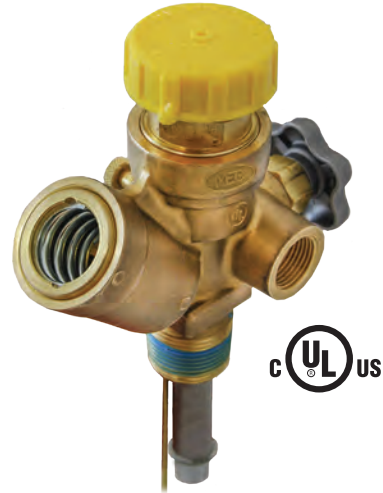
Válvula de múltiple servicio MES-PVE2035AT
